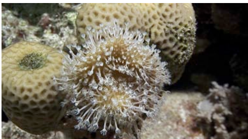
corall ( Goniopora sp.)
