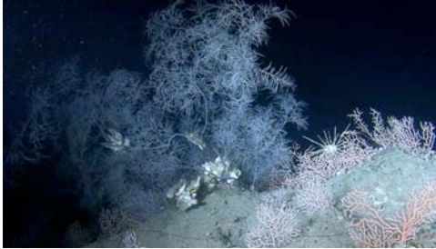
antipatari ( Antipathella subpinnata ) i gorgònia ( Eunicella sp.)
